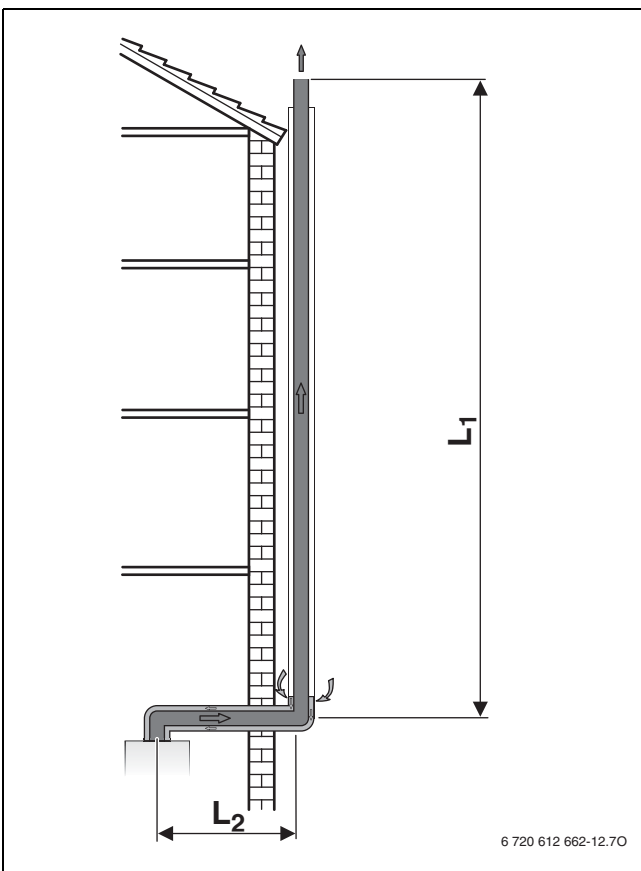
Fig. 16 Passaggio gas combustivi sulla facciata secondo C 53
