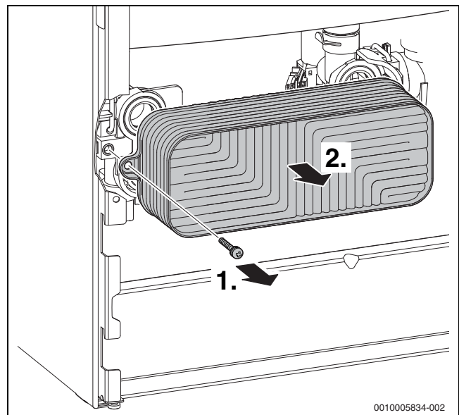
Fig. 60 Smontaggio dello scambiatore di calore a piastre
