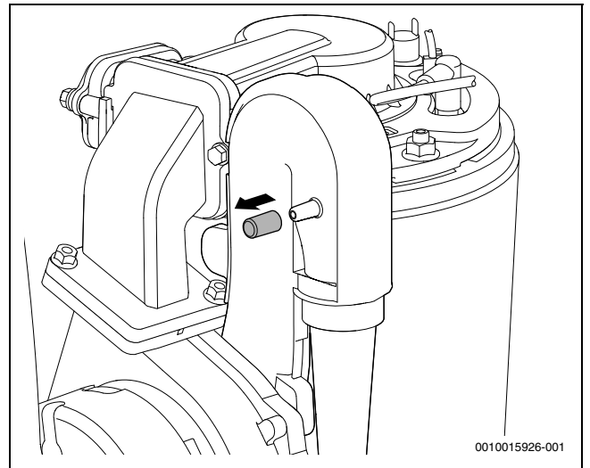
Fig. 42 Manicotto di misurazione sul miscelatore
