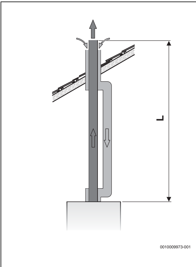
Fig. 15 Passaggio gas combustivi verticale secondo C 33
