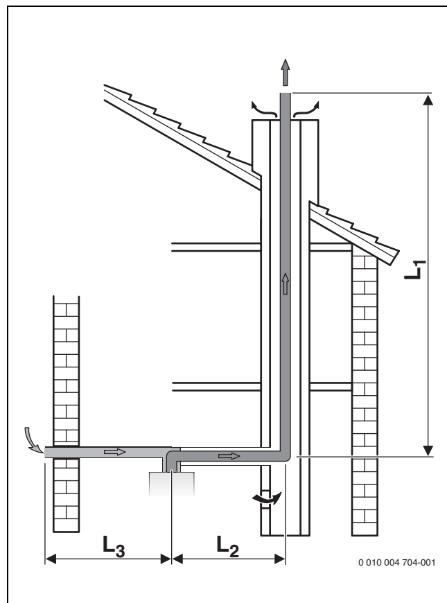
Fig. 10 Condotto di scarico combusto tramite cavedio secondo C 53
