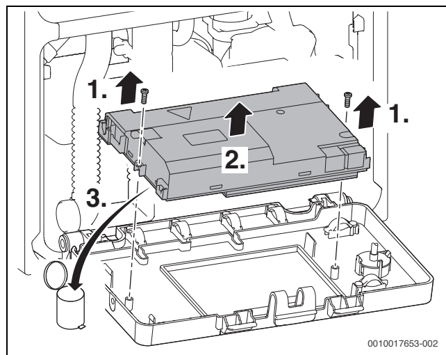
Fig. 68 Rimozione della copertura e sostituzione della scheda elettronica
