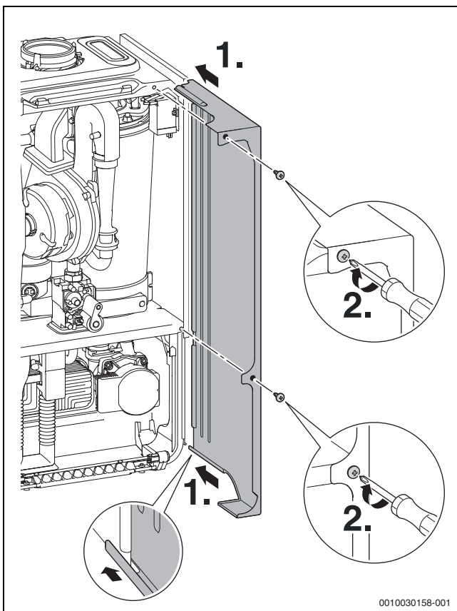
Fig. 70 Riapplicazione del rivestimento laterale
