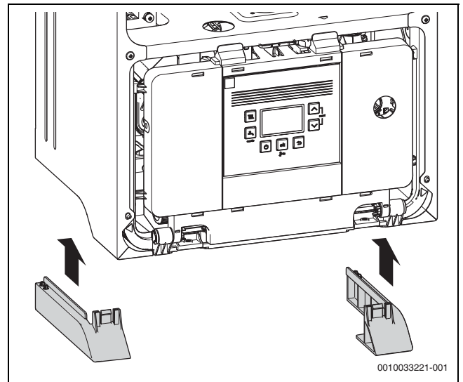
Fig. 71 Inserire strisce di plastica laterali
