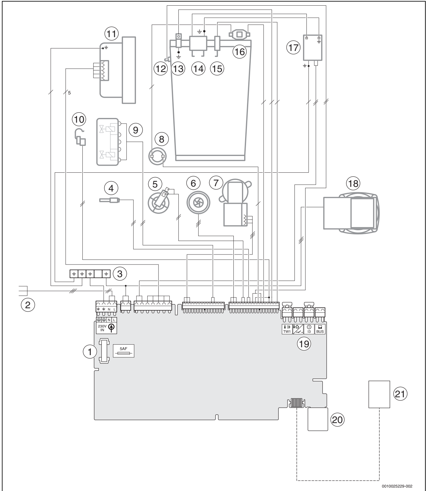
Fig. 73 Cablaggio elettrico
