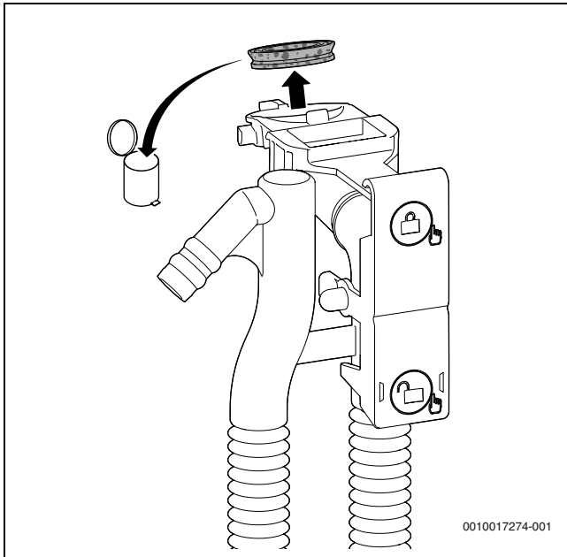
Fig. 54 Sostituzione della guarnizione posta sul lato superiore del sifone per la condensa
