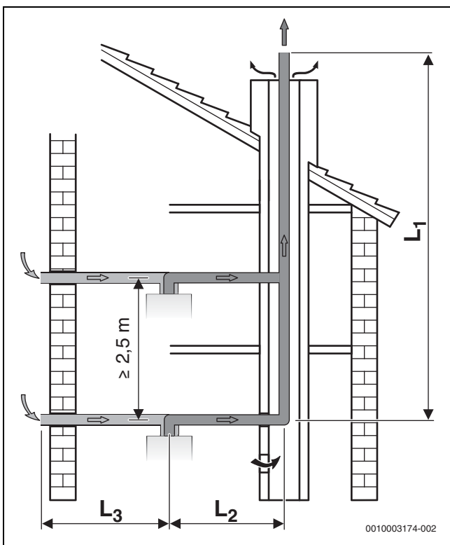
Fig. 19 Occupazione multipla con condotto aspirazione/scarico secondo C 83
